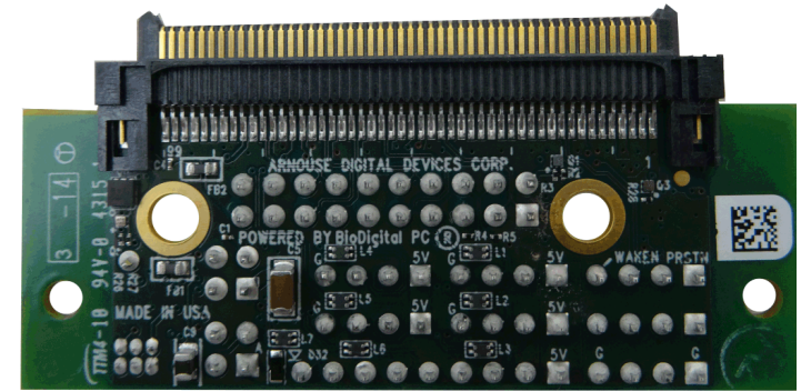
PCB BOTTOM
